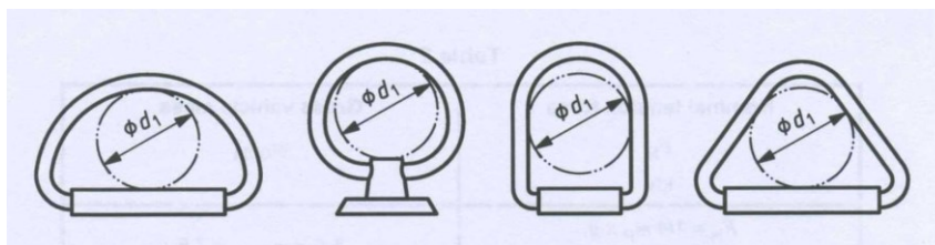
Rys. 2. Kształt elementów do mocowania ładunku.
