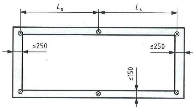
Rys. 1. Rozmieszczenie elementów do mocowania ładunku.
